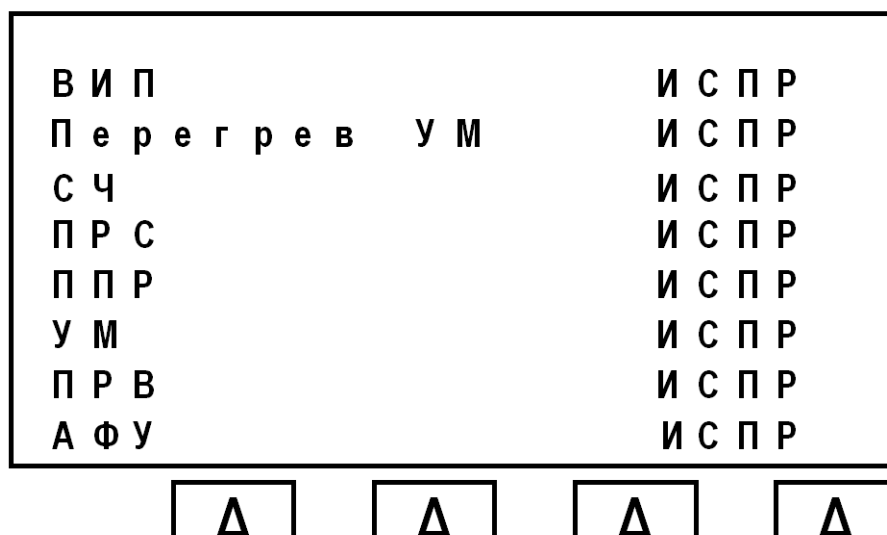
Рис. 10 Внешний вид результатов контроля
