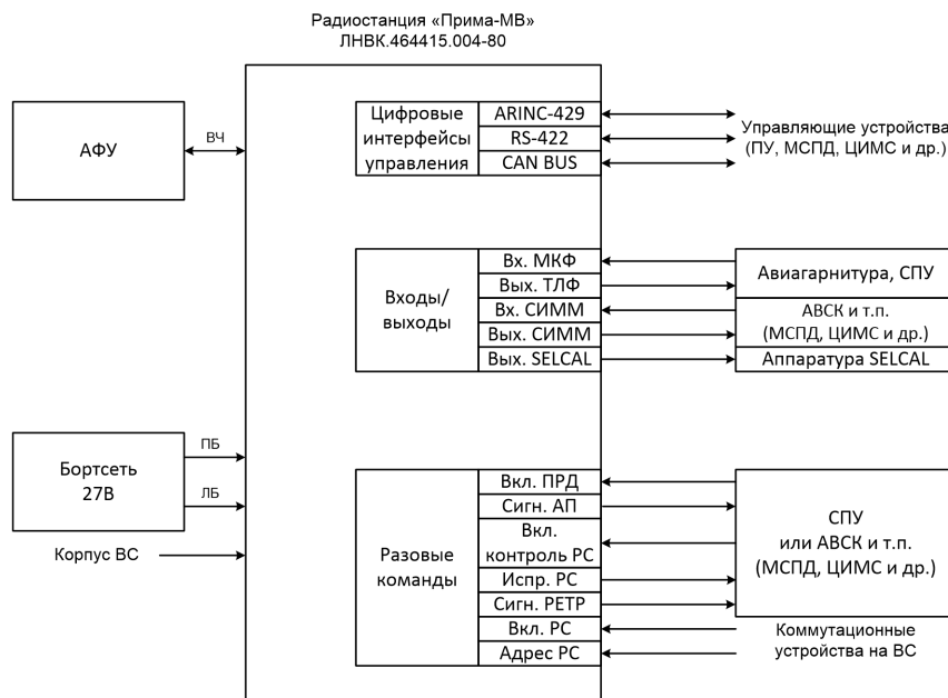
Рис. 1 Структурная схема подключения радиостанции
