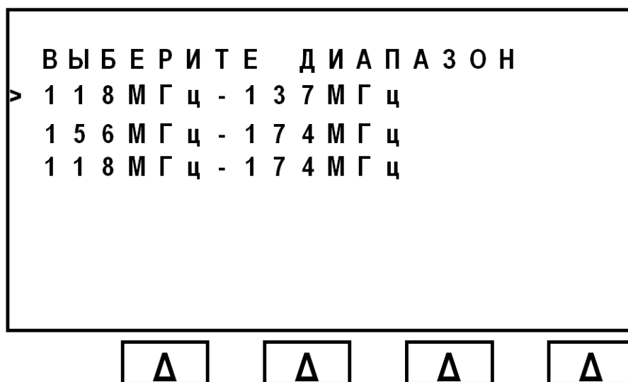
Рис. 9 Внешний вид страницы выбора диапазона контроля
