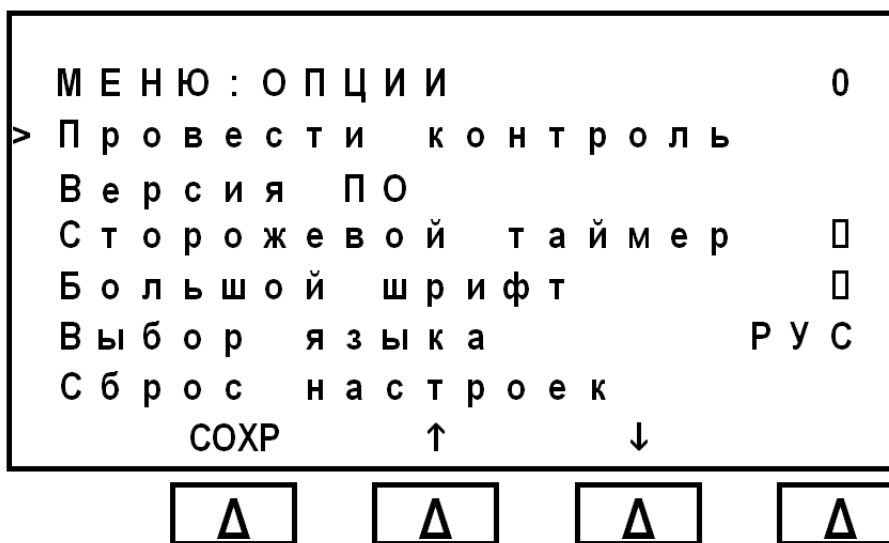
Рис. 6 Внешний вид страницы 0 меню режима настройки
