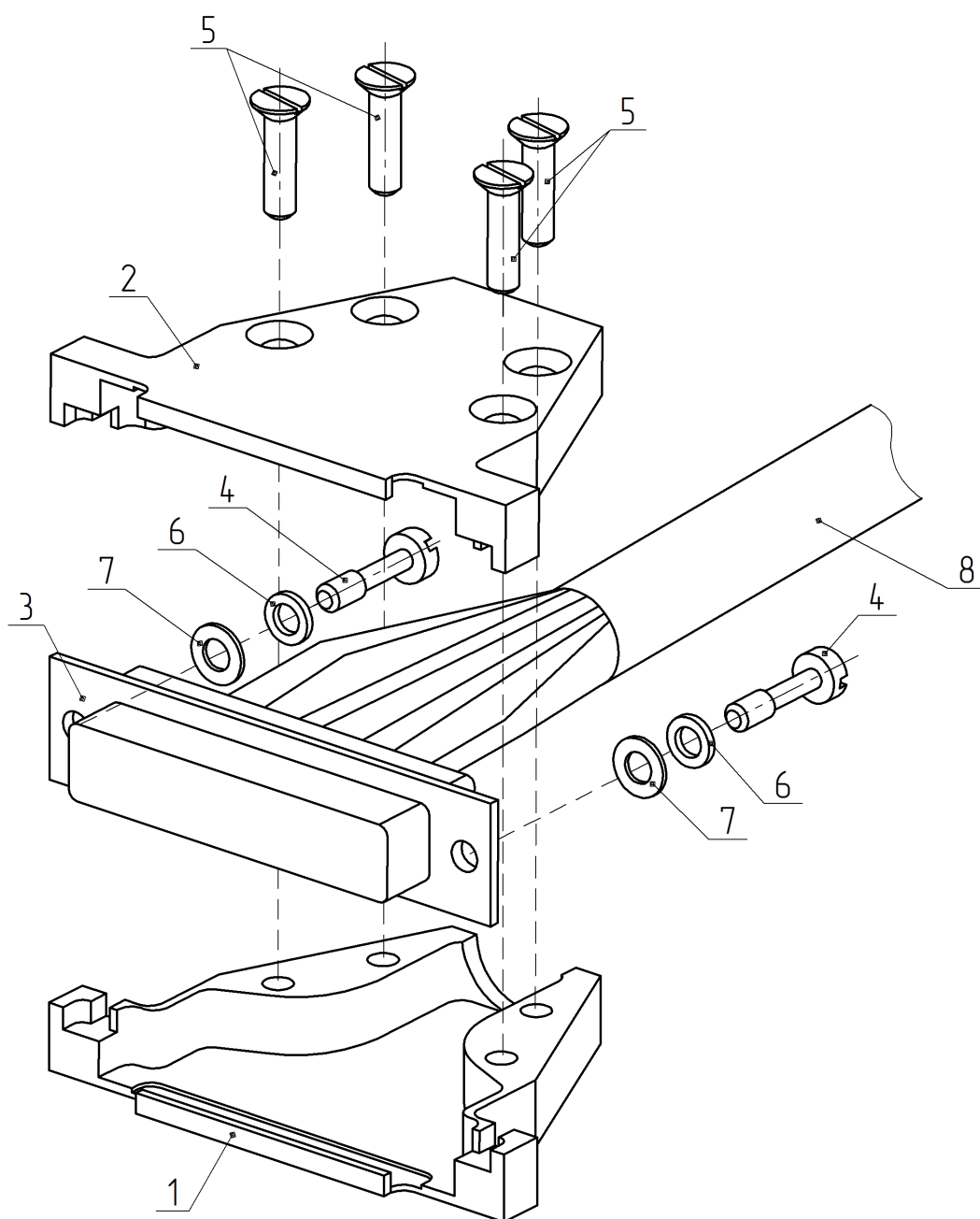
Рис. 1 Порядок сборки кожуха с соединителем
