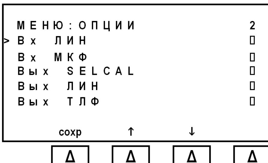
Рис. 8 Внешний вид страницы 2 меню режима настройки
